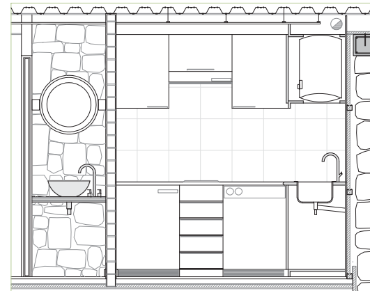
DETALLE TIPO COCINAS-ASEO (apartamentos de planta baja)
